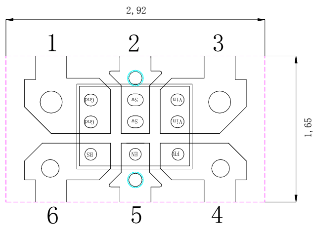
框架正面视图 Leadframe Top view ASM机台
